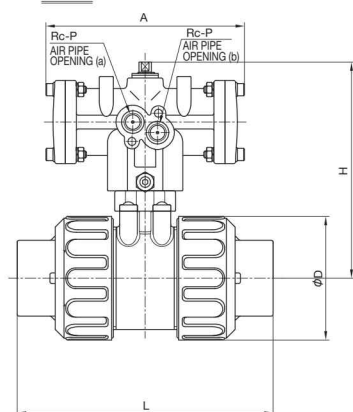
SOCKET
