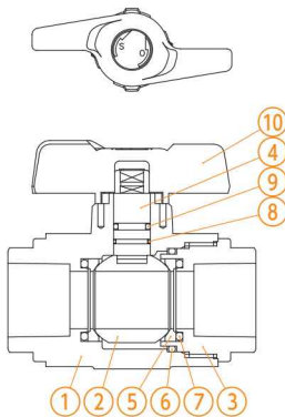
SOCKET
